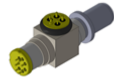
25G/50G PON ONU BOSA
