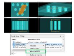
Ansys Lumerical
